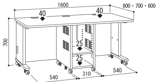
▲CAI-16XW寸法図
