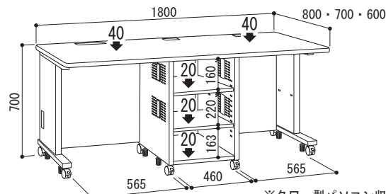
▲CAI-18XW寸法図
